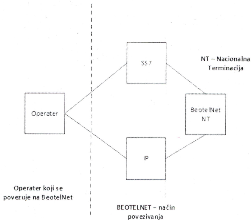
Slika 1. Mogućnosti povezivanja operatora na mrežu BeotelNet-a
